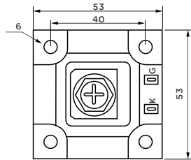
M**350-500A模块
