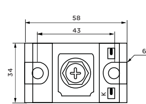
M**200-300A模块
