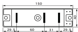
TM130-200A系列焊机专用模块
