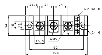
MT/D*110焊机专用模块A
