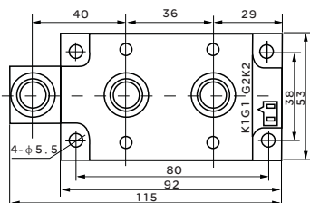
M** 200-300A系列模块
