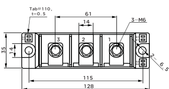
MT/D*150-300A系列焊机专用模块
