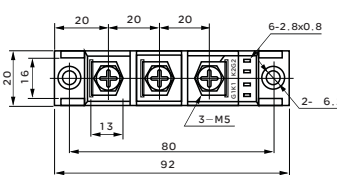
M** 25-110A模块
