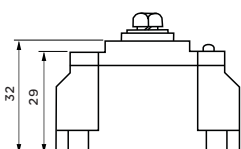
MT/D 100A模块
