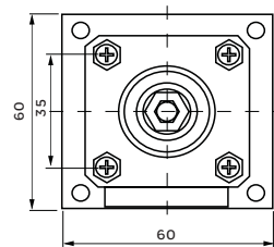
MP 25模块
