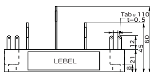
TM130-200A系列焊机专用模块
