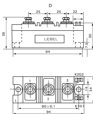
M** 130-160A系列模块
