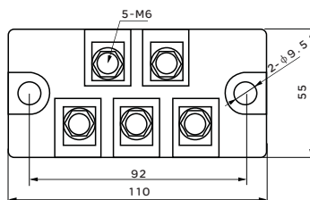
MDS 150-200A桥式模块
