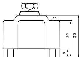
MT/D 200A模块
