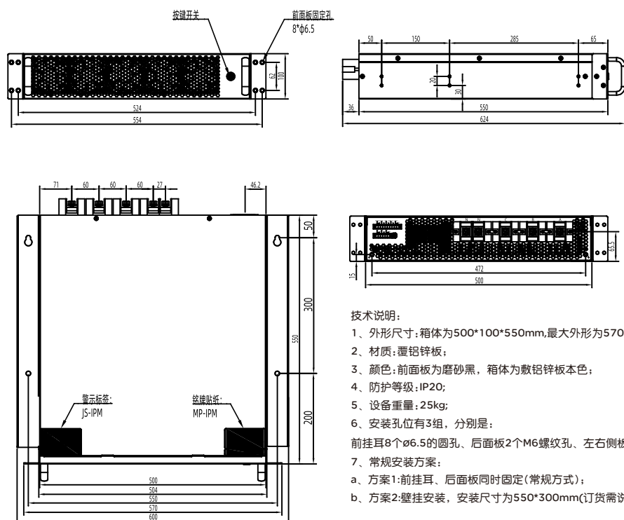
RD-PQC-APF/100、150A-0.4/4L-S外形尺寸图
