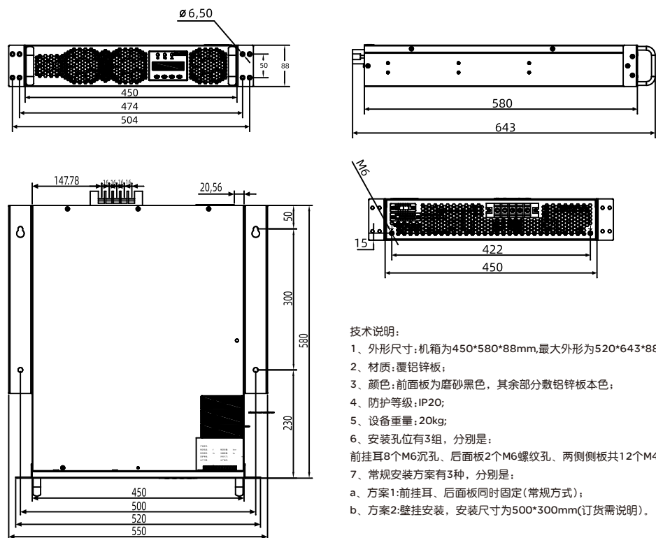
RD-PQC-APF/50A-0.4/4L-N外形尺寸图
