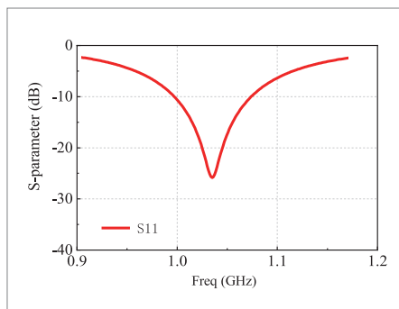
天线反射系数
