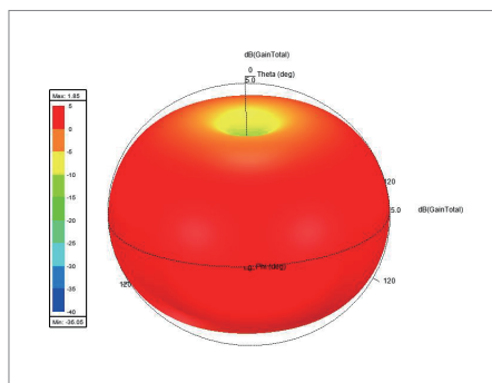
天线 3D 辐射方向图
